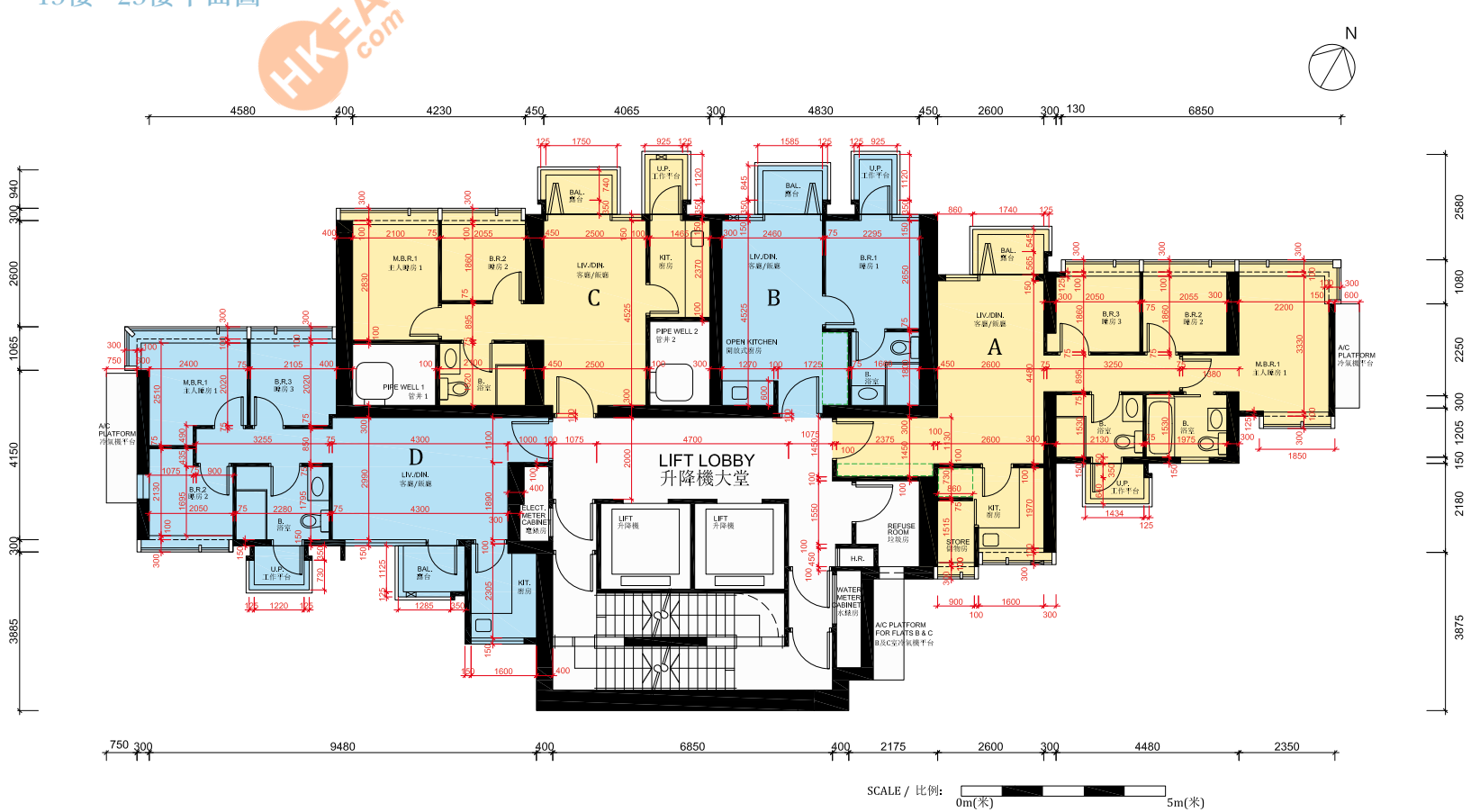
15/F - 23/F Floor Plan 15樓 - 23樓平面圖
