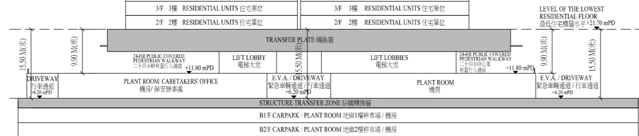
CROSS - SECTION PLAN C 橫截面圖 C
