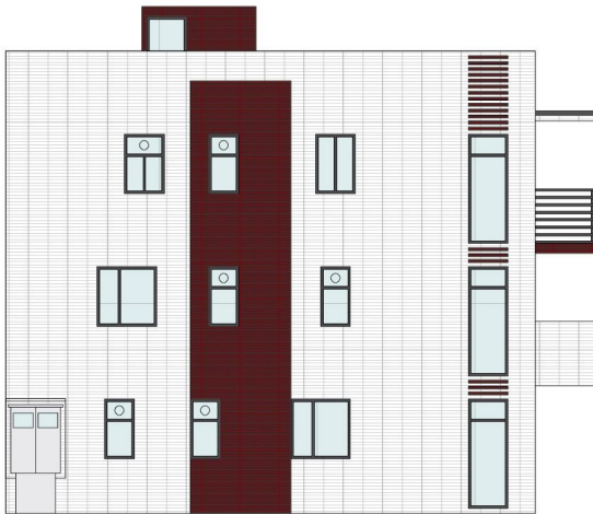
ELEVATION 3 立面圖三 WEST
