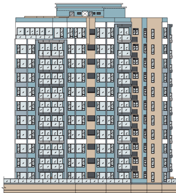
Elevation 2 立面 2
