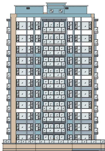
Elevation 1 立面 1
