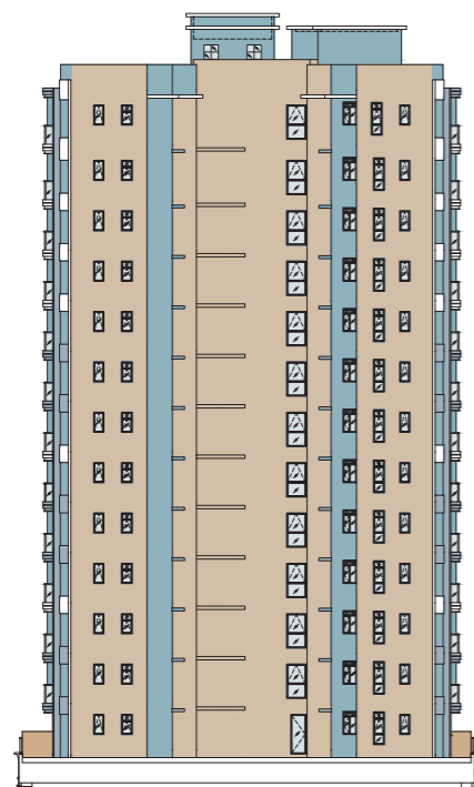
Elevation 3 立面 3
