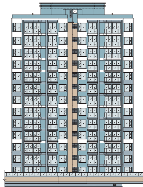
Elevation 4 立面 4
