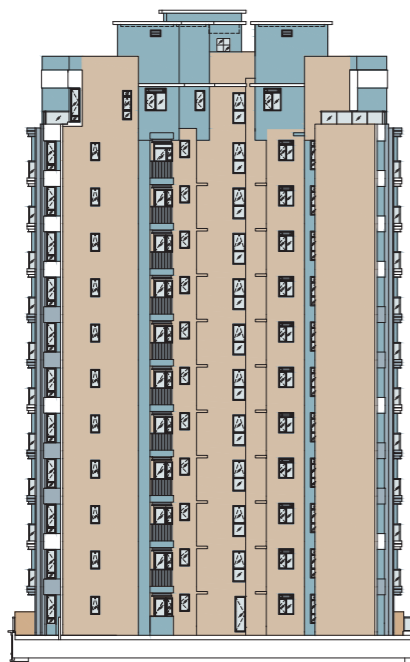
Elevation 3 立面 3
