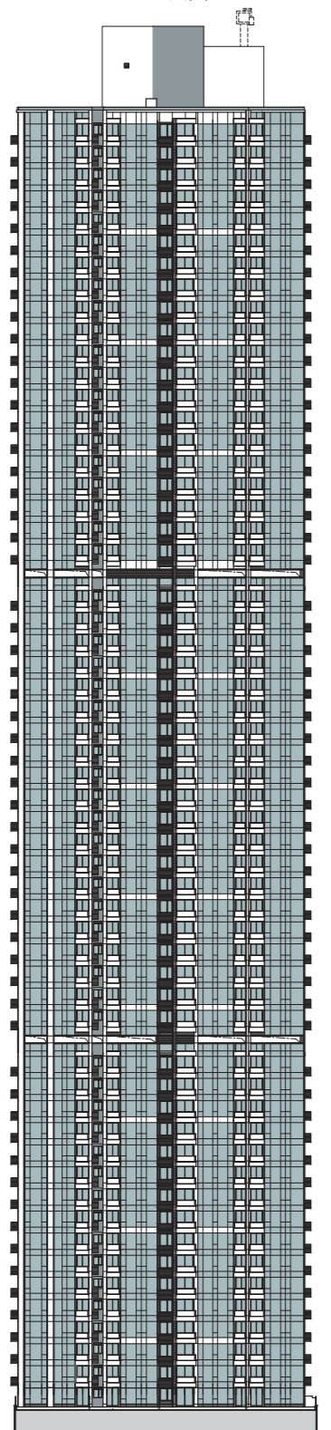
Elevation B1 立面圖 B1
