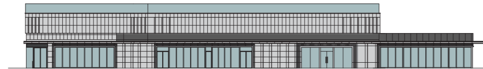
Podium Roof Elevation E1 平台天台立面圖 E1
