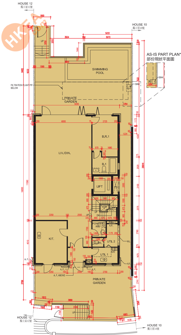
G/F FLOOR PLAN 地下平面圖
