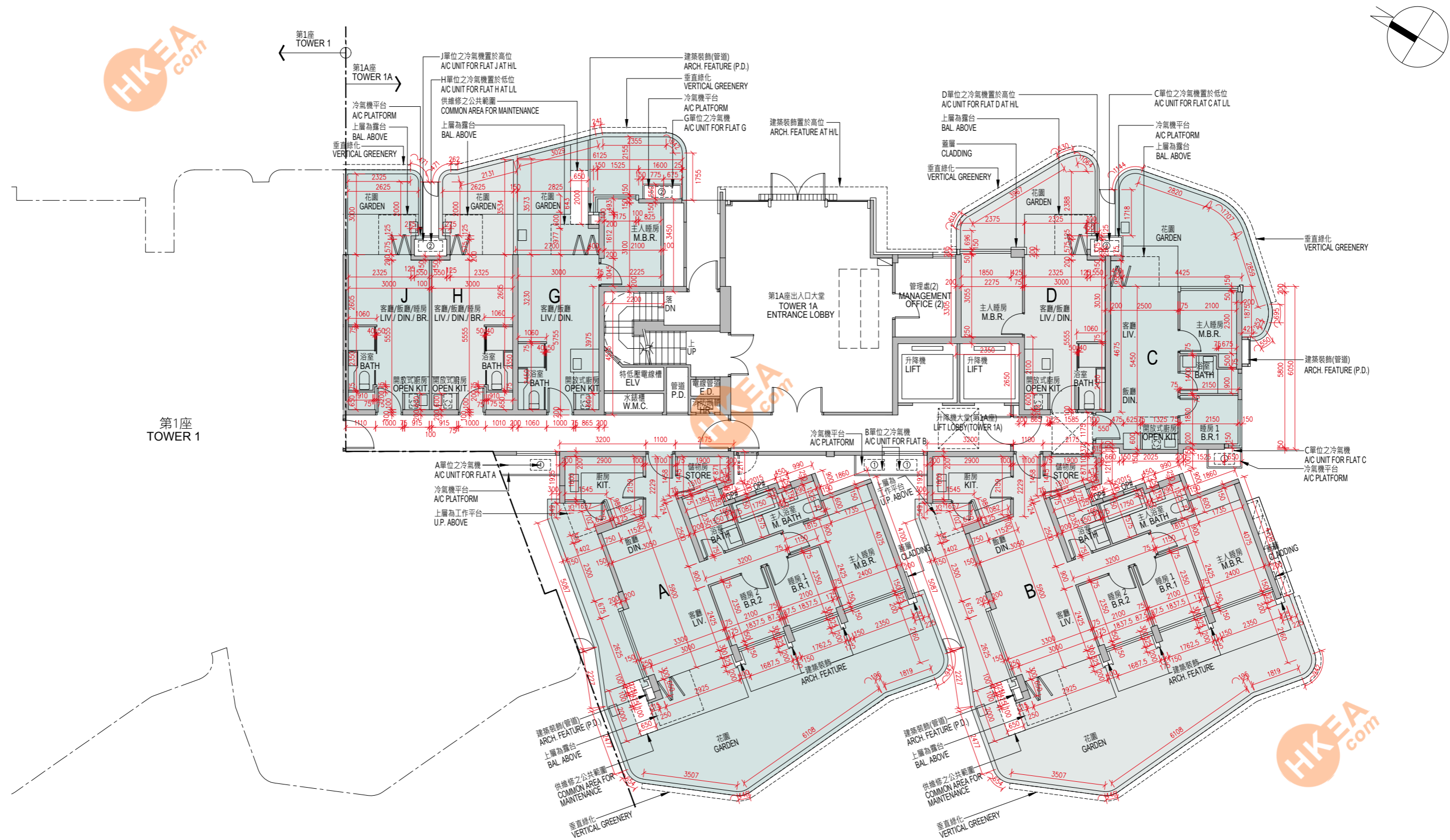
第1A座 TOWER 1A 地下平面圖 G/F PLAN
