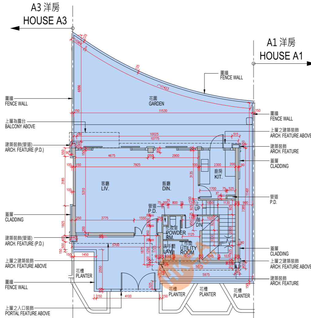
地下平面圖 G/F PLAN
