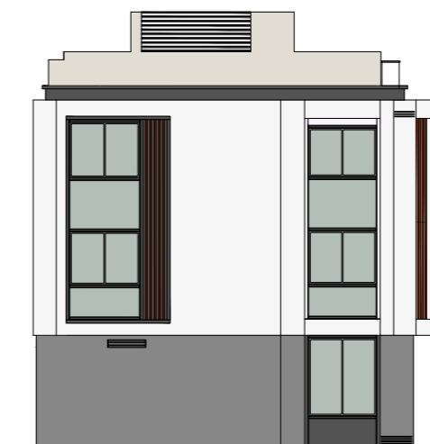
立面圖 D1 (適用於 B12 洋房) Elevation Plan D1 For House B12)
