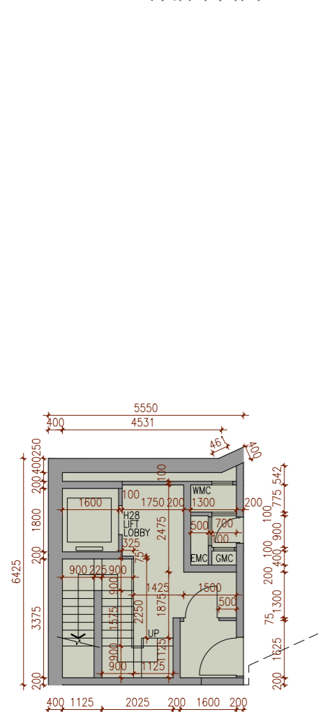
BASEMENT FLOOR PLAN 地庫層平面圖
