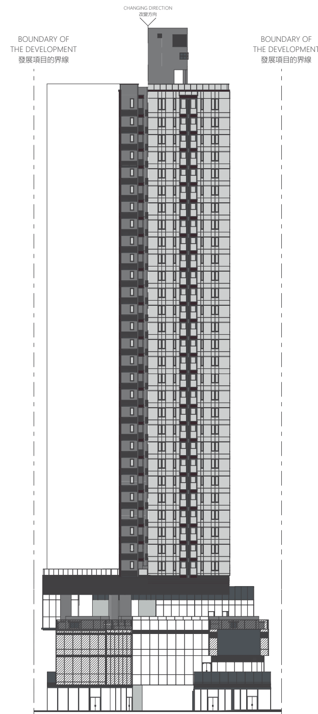
Elevation Plan B 立面圖 B
