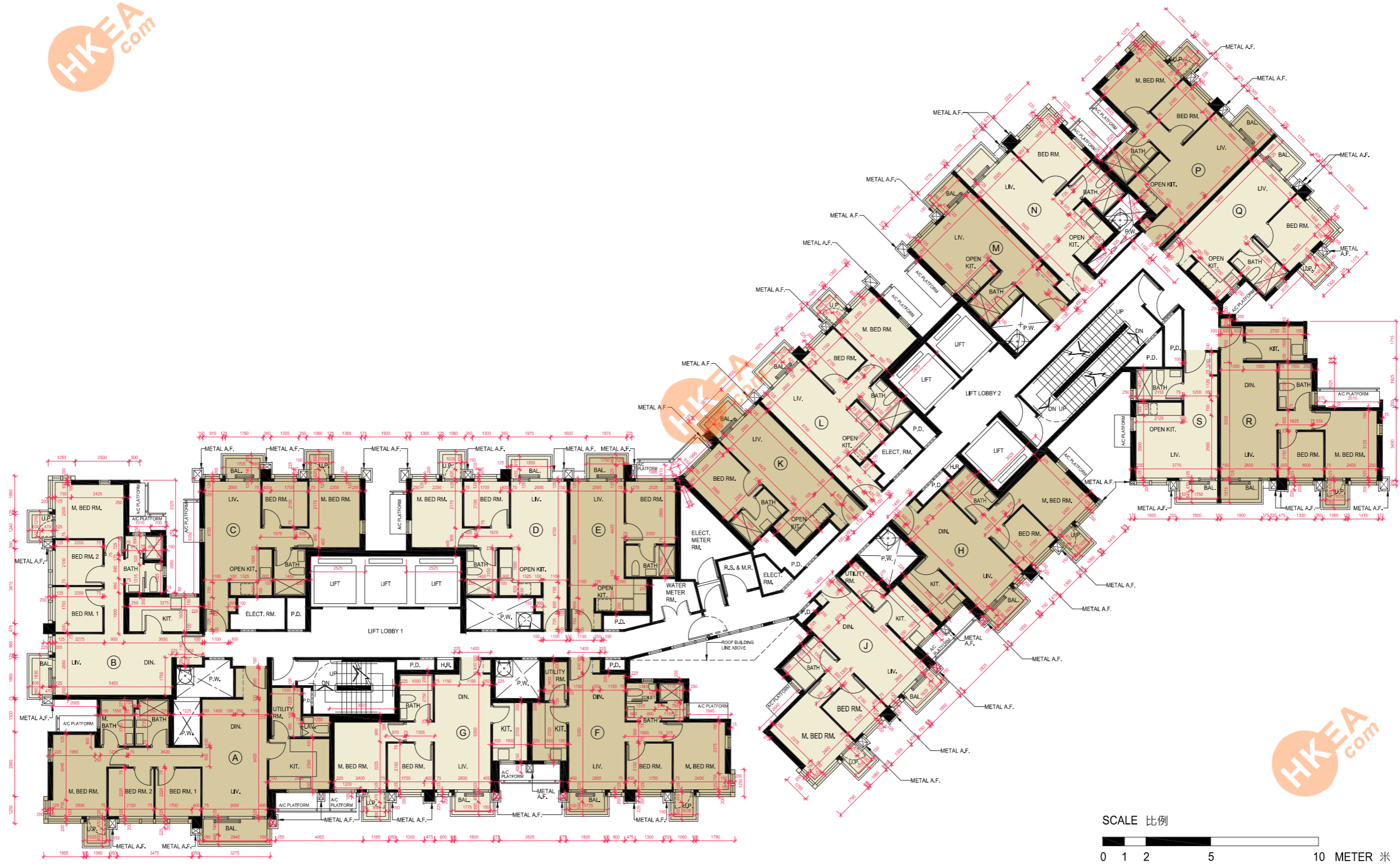
33/F Floor Plan 33樓樓面平面圖
