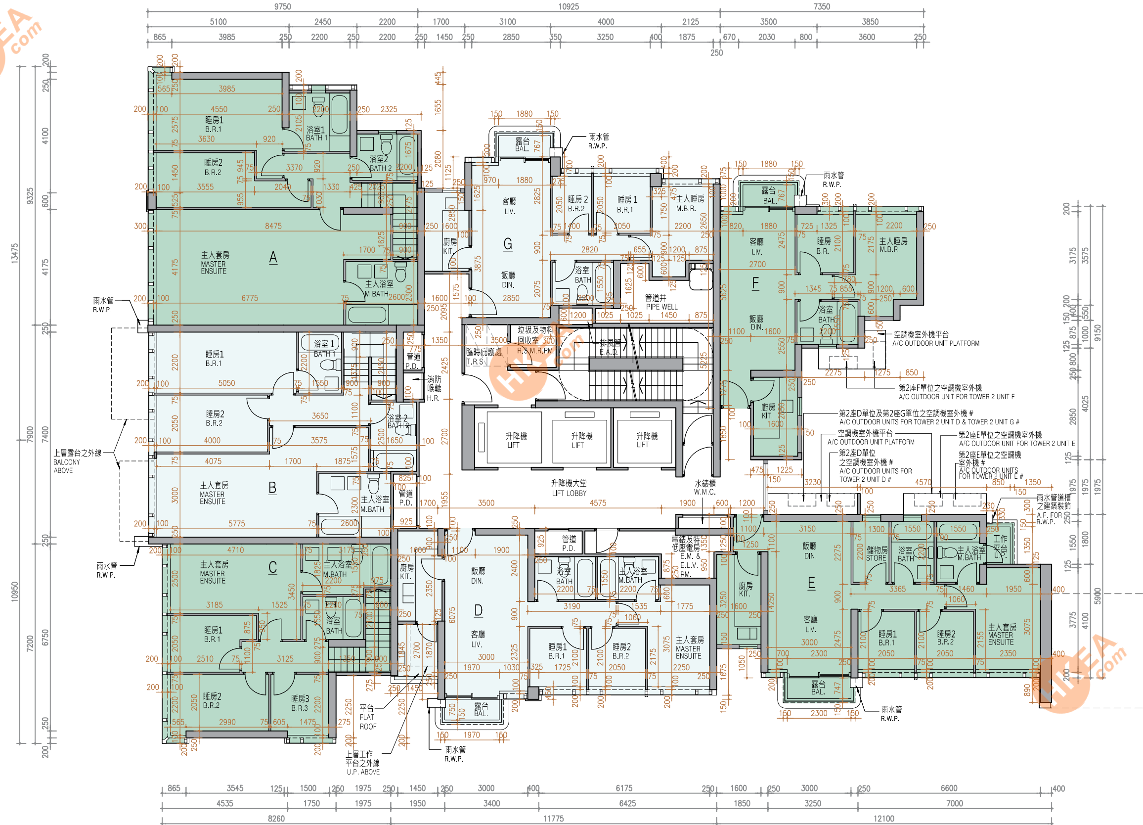
TOWER 2 2/F FLOOR PLAN 第2座 2樓 樓面平面圖
