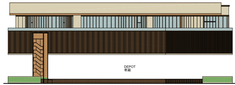
ELEVATION B 立面圖 B
