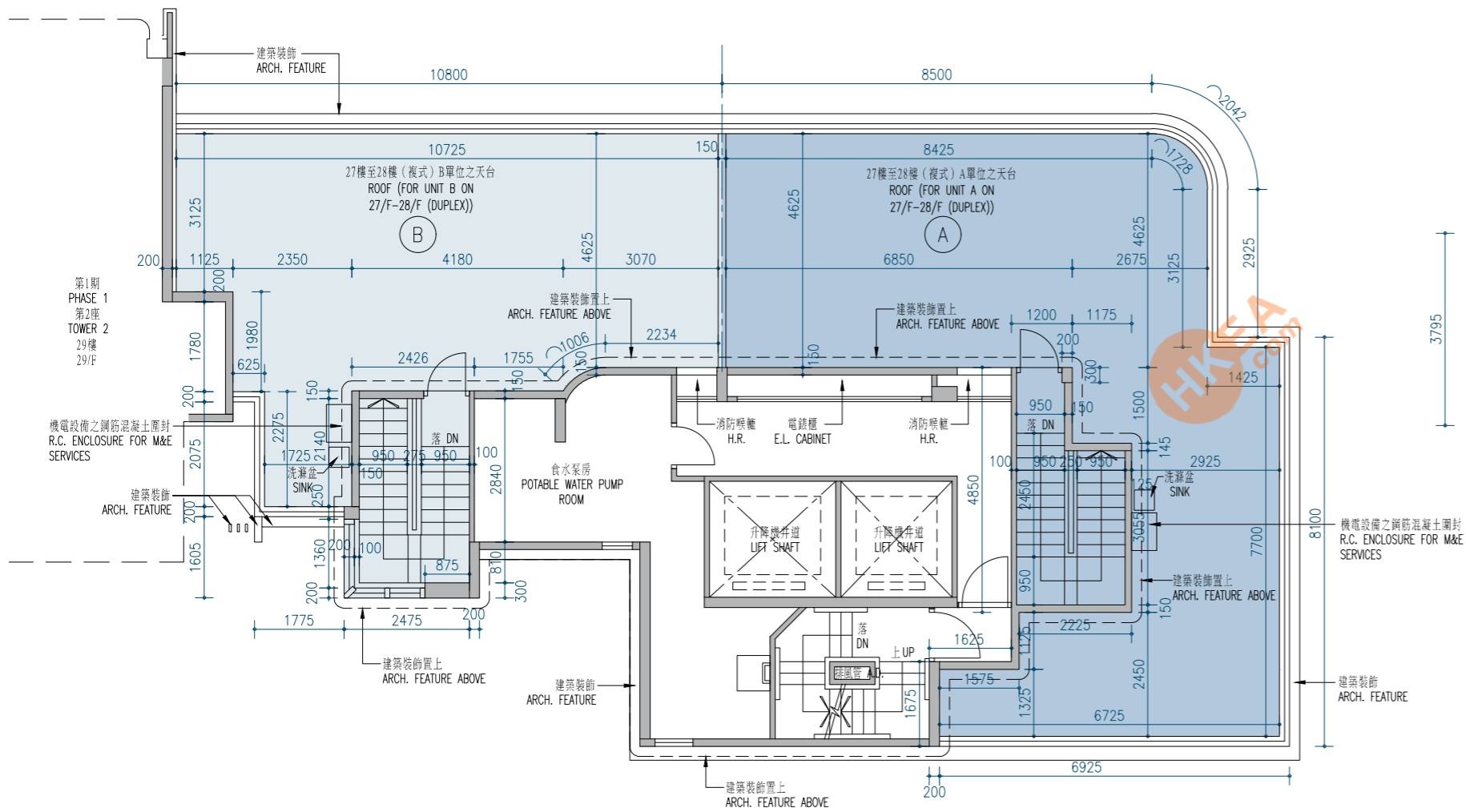
Roof Plan 天台平面圖
