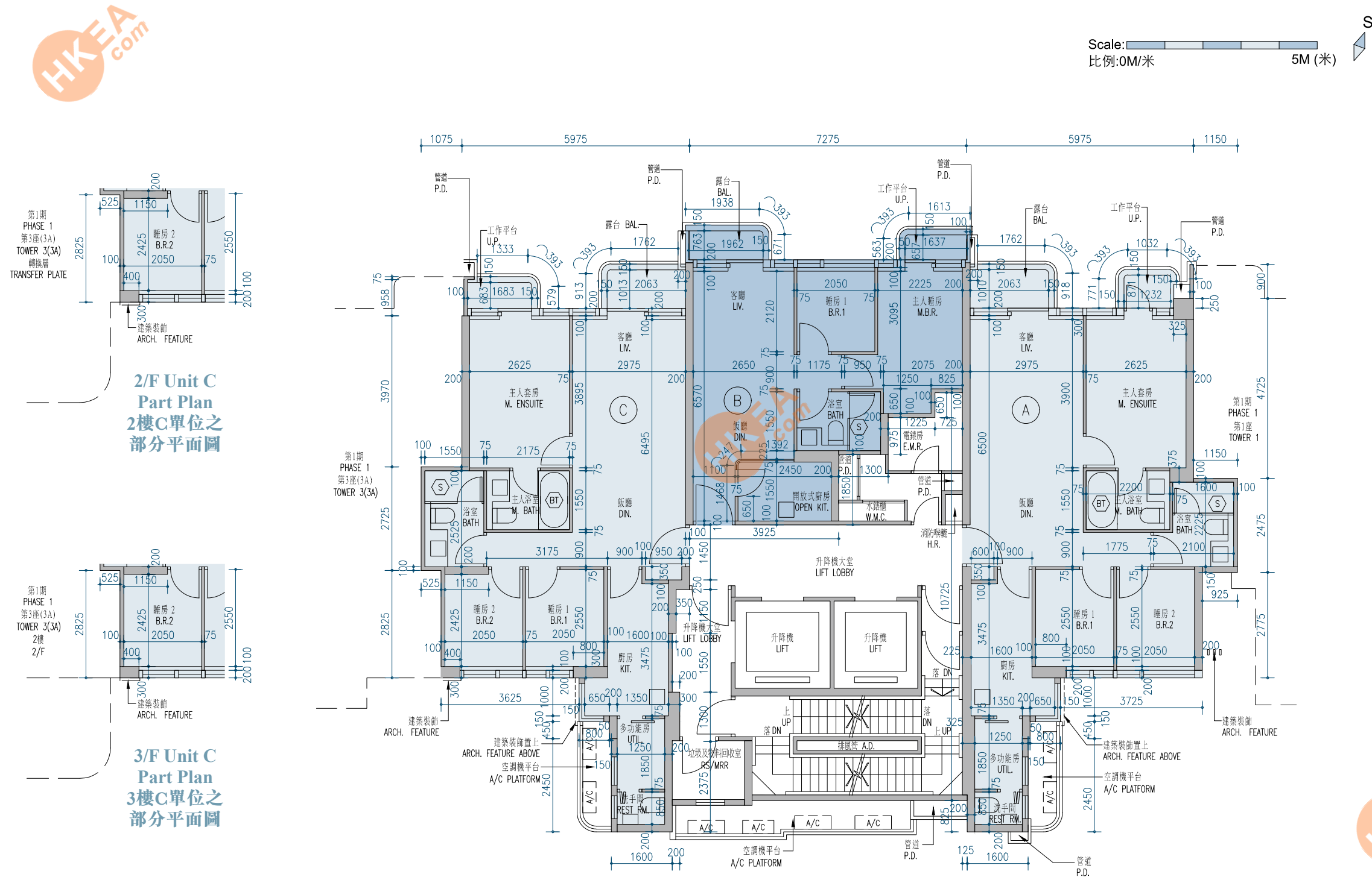
Phase 1 Tower 2 2/F-3/F, 5/F-12/F, 15/F-17/F, 19/F-23/F, 25/F-26/F Floor Plan 第1期 第2座2樓至3樓、5樓至12樓、15樓至17樓、19樓至23樓、25樓至26樓樓面平面圖
