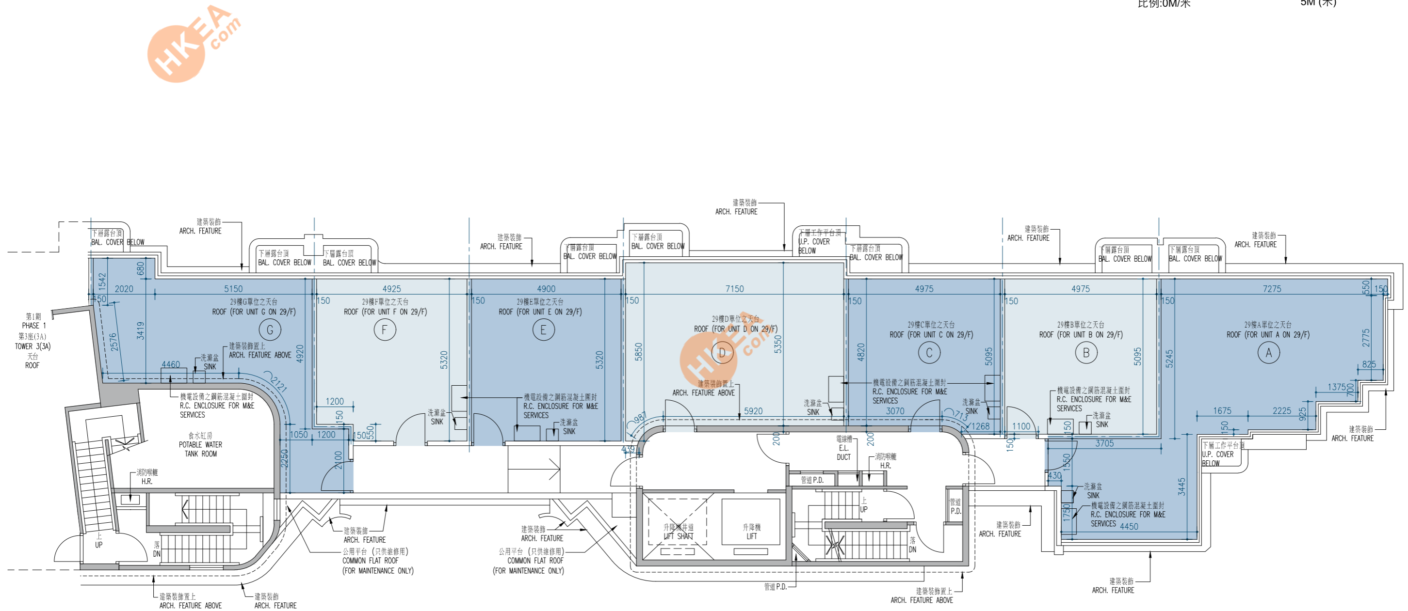
Phase 1 Tower 3(3B) Roof Floor Plan 第1期 第3座(3B) 天台樓面平面圖
