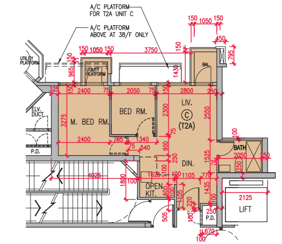
Part Plan of Tower 2 (2A) Unit C on 38/F 第2座(2A)38樓C單位部份圖
