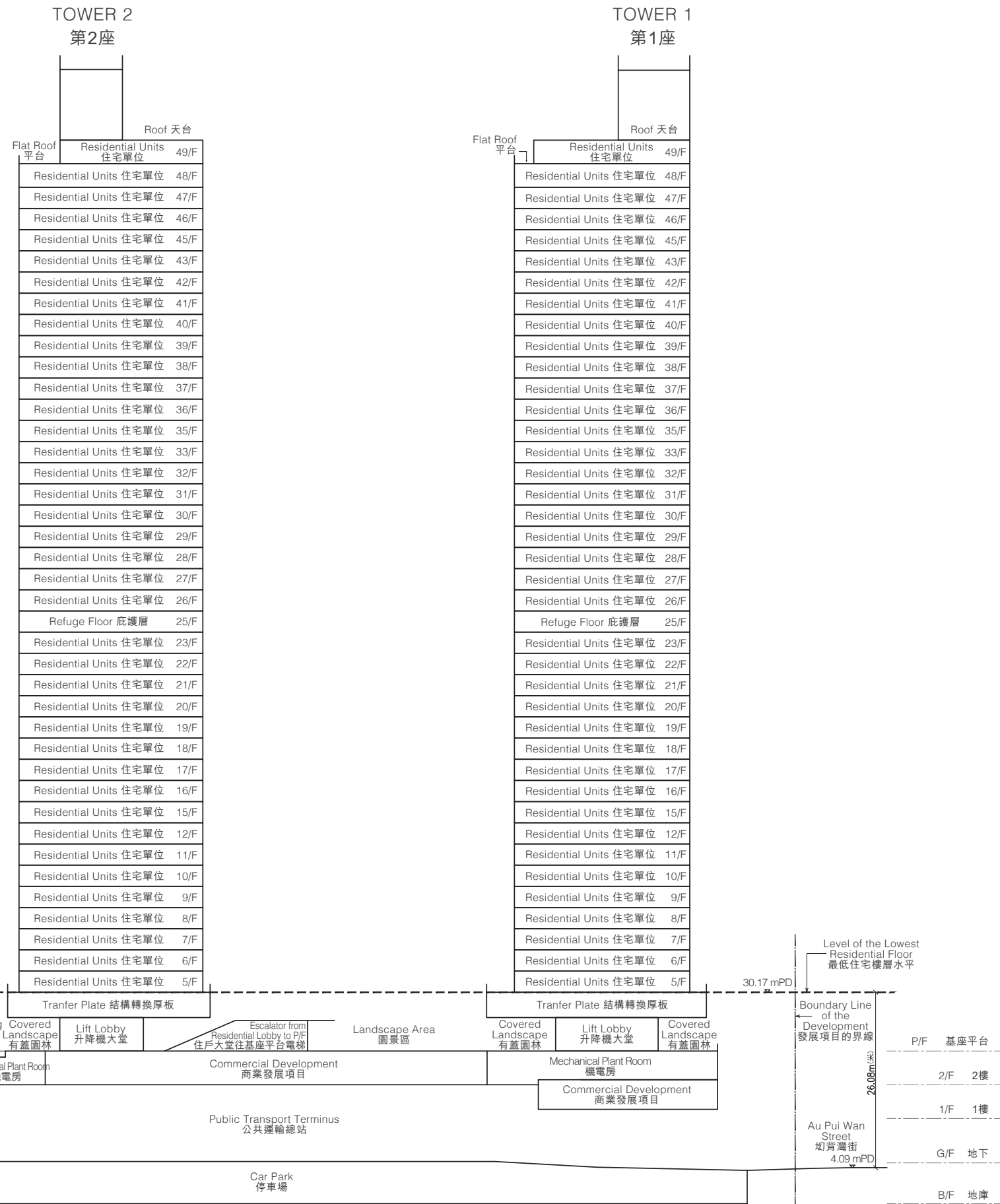
CROSS-SECTION A-A 橫截面圖 A-A
