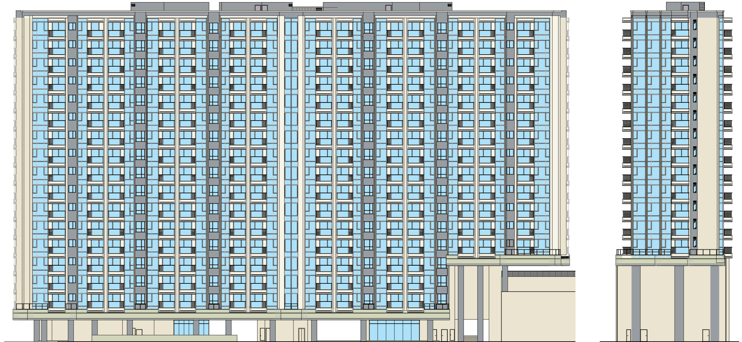
Elevation A 立面圖 A
