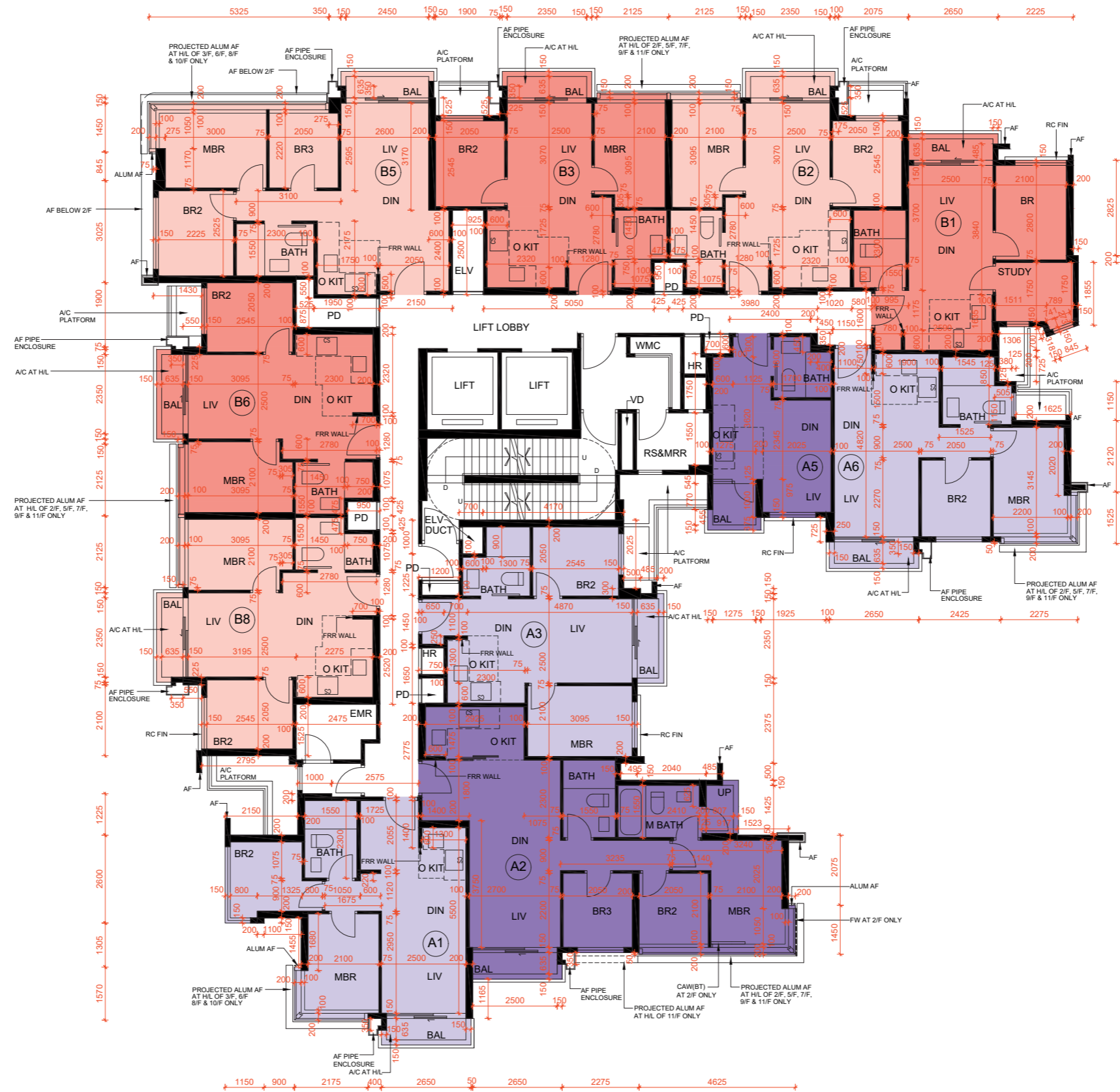
GREENWOOD TOWER 5 2/F-3/F AND 5/F-11/F FLOOR PLAN 翠景閣第5座 2樓至3樓 及 5樓至11樓平面圖
