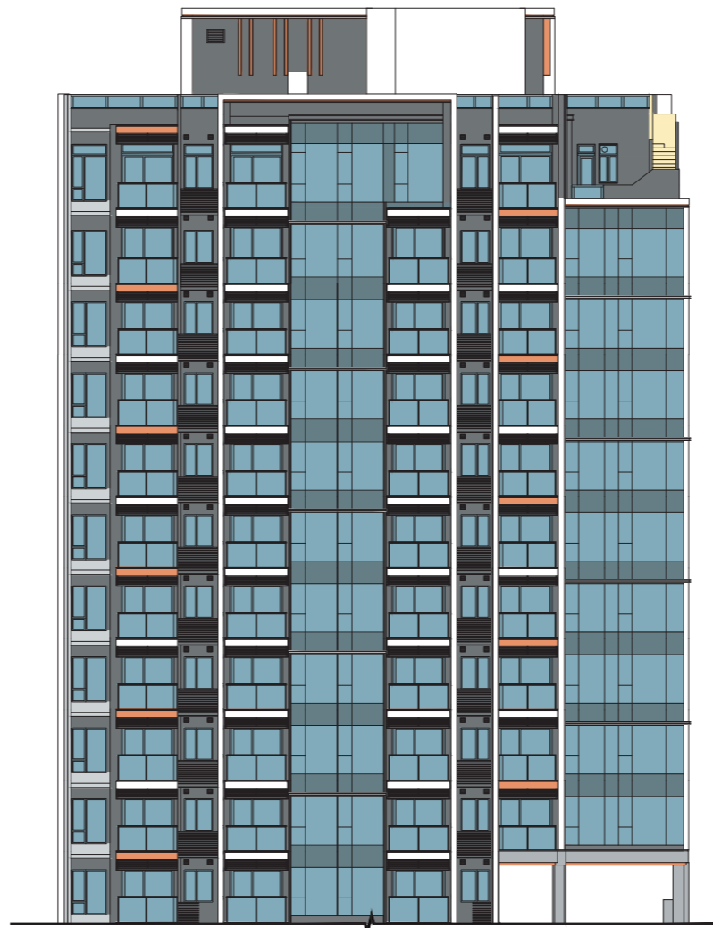
ELEVATION 4 立面 4
