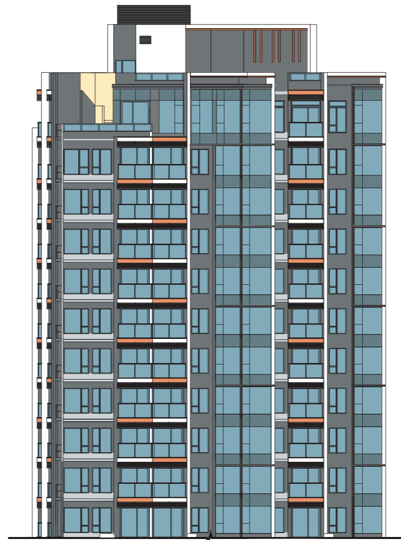
ELEVATION 2 立面 2
